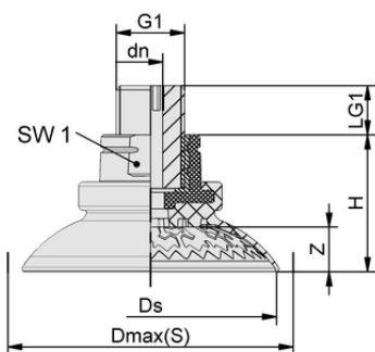
Données de construction SAX 50 ED-85 M10-AG
