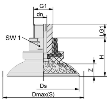
デザインデータ SAX 40 ED-85 G3/8-AG
