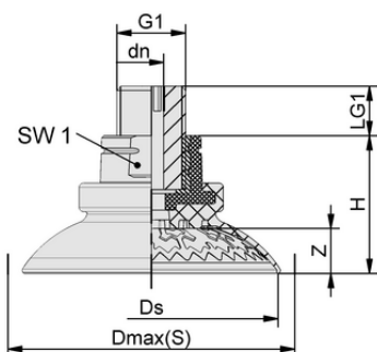
Données de construction SAX 115 ED-85 G3/8-AG
