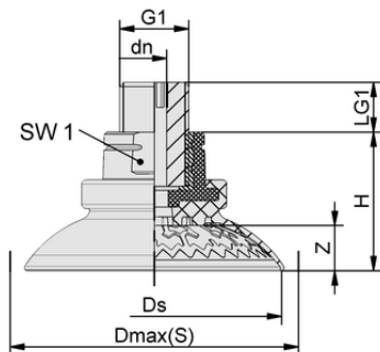
Données de construction SAX 50 ED-85 G1/4-AG
