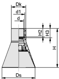
Dati di costruzione SVE 53 PU-55 SC080
