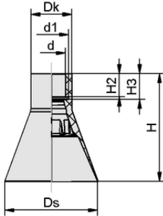
Tasarım verileri SVE 53 PU-55 SC080
