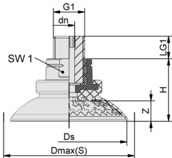
Dati di costruzione SAX 80 ED-85 M10-AG RP
