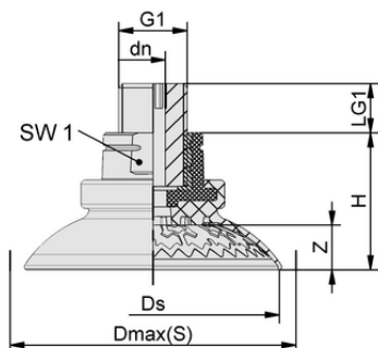
デザインデータ SAX 80 ED-85 M10-AG RP
