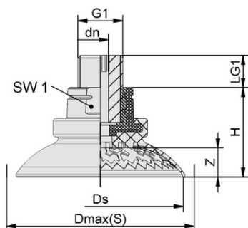
Конструктивные данные SAX 115 ED-85 G1/4-AG
