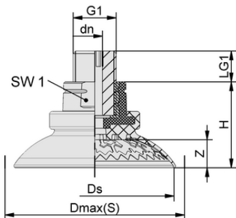
Конструктивные данные SAX 30 ED-85 G1/4-AG
