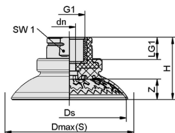
デザインデータ SAX 100 ED-85 G3/8-IG
