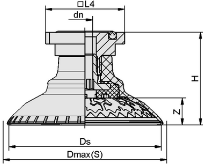
Tasarım verileri SAXM 20 ED-85 RA
