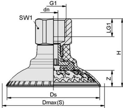
Tasarım verileri SAXM 20 ED-85 G1/4-IG
