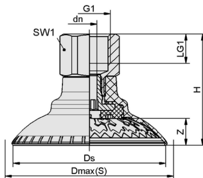
デザインデータ SAXM 20 ED-85 G1/4-IG
