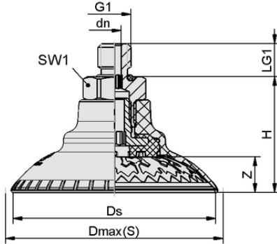
Tasarım verileri SAXM 115 ED-85 G1/4-AG
