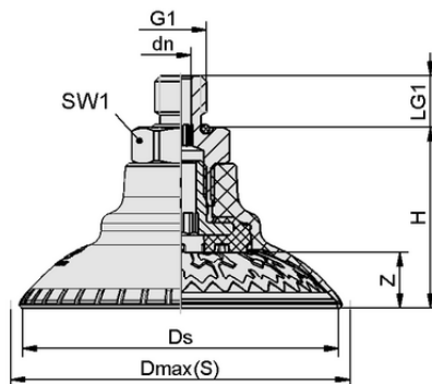
デザインデータ SAXM 100 ED-85 G3/8-AG
