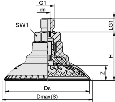
Tasarım verileri SAXM 100 ED-85 G1/4-AG
