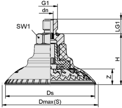
Tasarım verileri SAXM 80 ED-85 G3/8-AG
