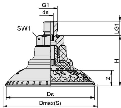
デザインデータ SAXM 40 ED-85 G1/4-AG
