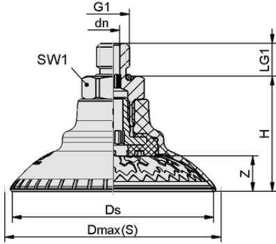
Tasarım verileri SAXM 40 ED-85 G1/4-AG
