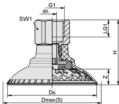
デザインデータ SAXM 100 ED-85 G3/8-IG
