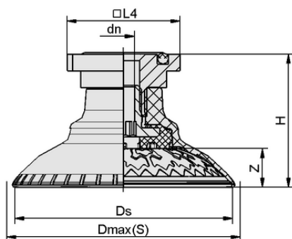
デザインデータ SAXM 60 ED-85 RA
