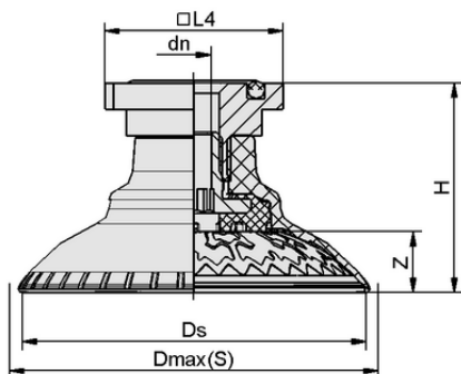
Dati di costruzione SAXM 60 ED-85 RA
