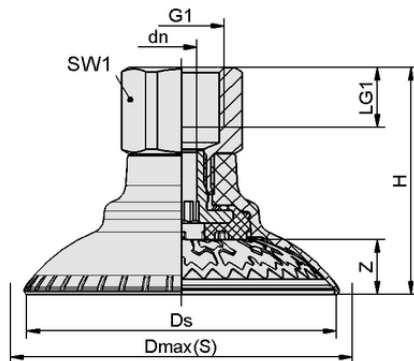
デザインデータ SAXM 50 ED-85 G3/8-IG
