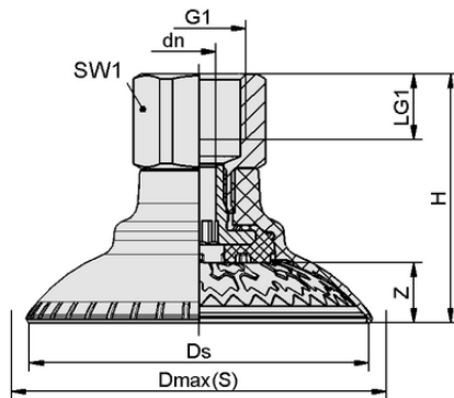
デザインデータ SAXM 40 ED-85 G3/8-IG
