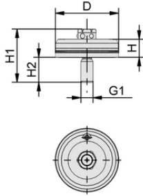
Tasarım verileri SQC-MB-62.9x18-M12-AG
