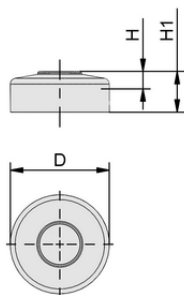
Конструктивные данные ABDK 68x12 SQC
