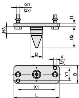
Konstruktionsdaten GR-E SGM-HPm 30 CP9.6 SET
