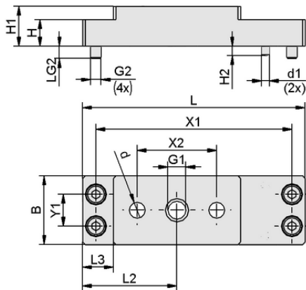
デザインデータ HTS-AE SGM-HPm 30/40 OP MS
