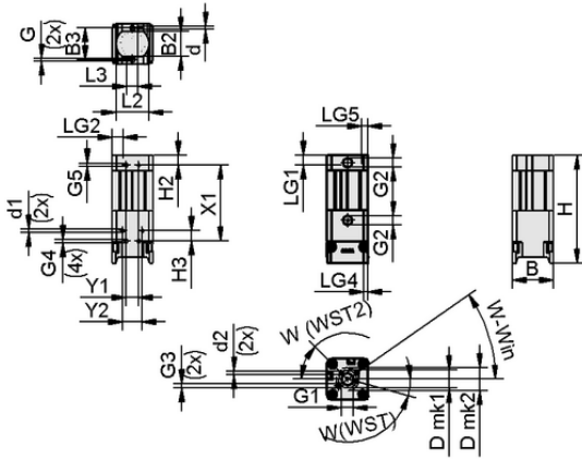
Tasarım verileri SGM-HPm 30 G1/8-IG
