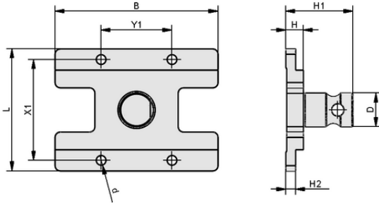
Tasarım verileri HTS-A2 SGM-HP 40x121 OP
