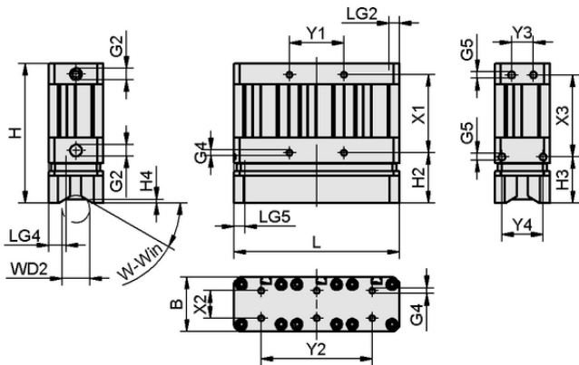
Dati di costruzione SGM-HP 40x121
