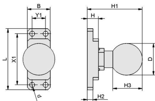
Datos de diseño HTS-A5 SGM-HP 50 OP
