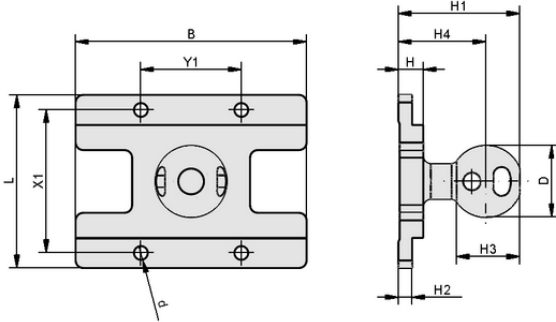
Tasarım verileri HTS-A5 SGM-HP 40x121 OP
