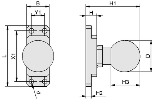
Tasarım verileri HTS-A3 SGM-HP 30/40 OP
