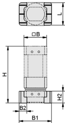
Konstruktionsdaten SCHUTZ SGM-30 ST
