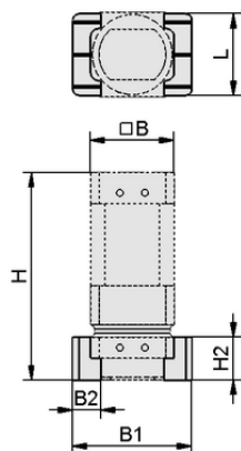
Konstruktionsdaten SCHUTZ SGM-40 ST
