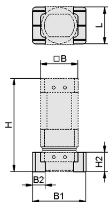
デザインデータ SCHUTZ SGM-50 ST
