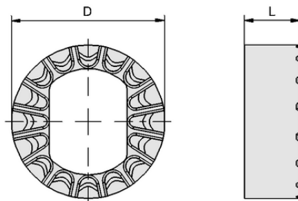
デザインデータ REIB-RING SGM-HT-HP 40 HT2-65
