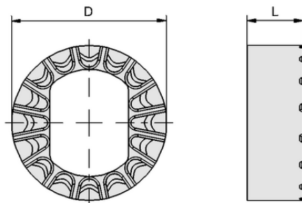
デザインデータ REIB-RING SGM-HT-HP 30 HT2-65
