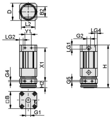
デザインデータ SGM-HT-HP 40 G1/4-IG
