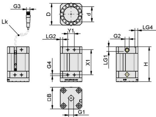
Datos de diseño SGM-HD-S 40 G1/4-IG PNP
