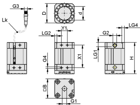
Dati di costruzione SGM-HD-S 40 G1/4-IG PNP
