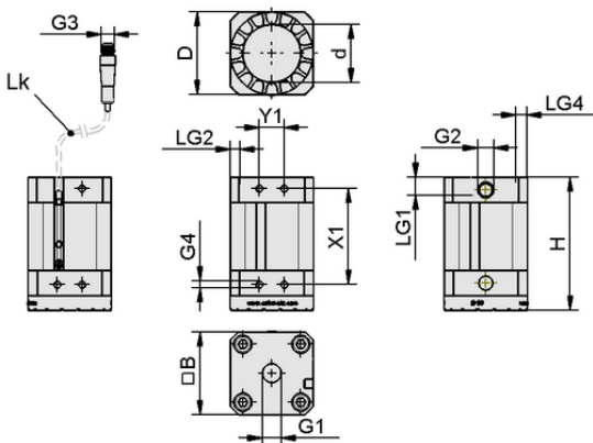
デザインデータ SGM-HD-S 40 G1/4-IG PNP
