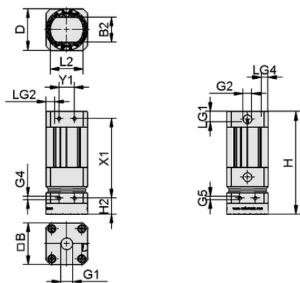
デザインデータ SGM-HP 50 G1/4-IG
