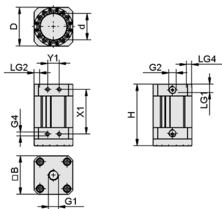
Données de construction SGM-HD 50 G1/4-IG
