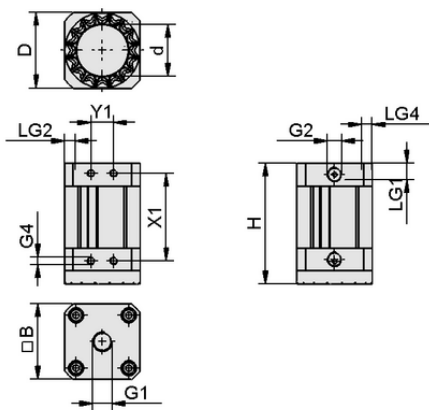
Dati di costruzione SGM-HD 70 G1/4-IG
