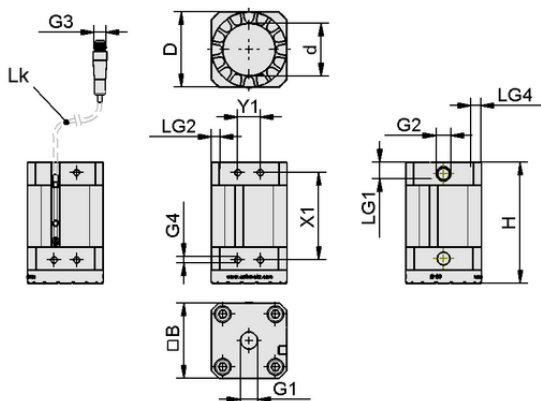
デザインデータ SGM-S 50 G1/4-IG PNP
