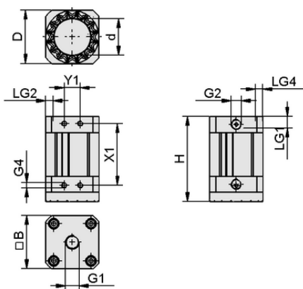
Datos de diseño SGM 50 G1/4-IG
