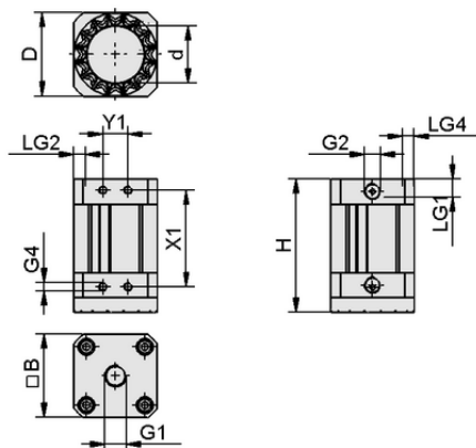
デザインデータ SGM 40 G1/4-IG
